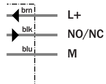
3 x 0.15 mm²
